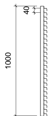
Corte esc. 1/20
