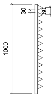
Corte esc. 1/20
